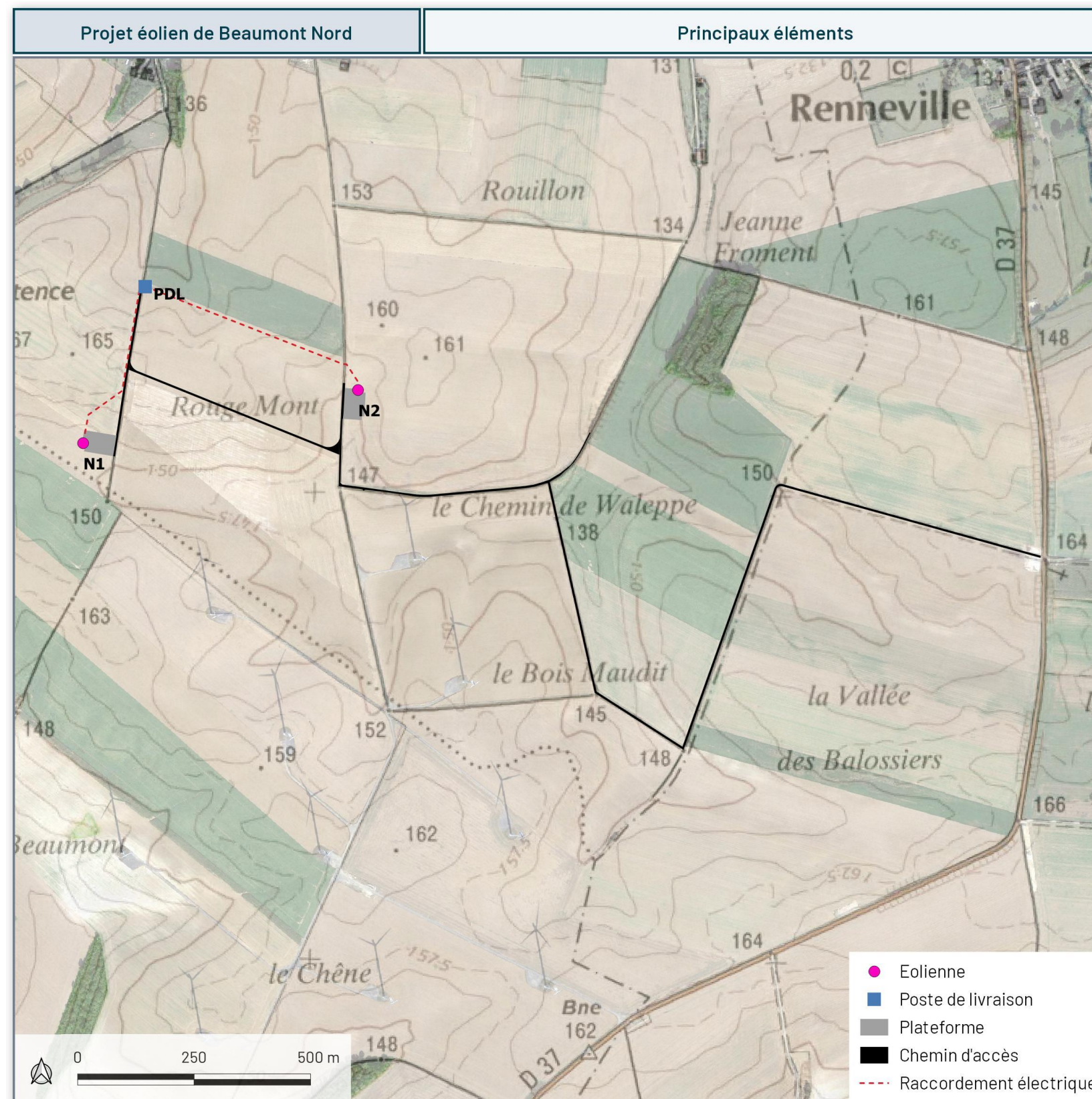
Carte 3 : Carte de localisation des principaux éléments du projet éolien de Beaumont Nord
